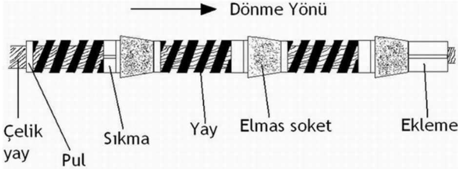
Şekil 1.1: Elmas teli oluşturan parçalar ve dizilişleri
